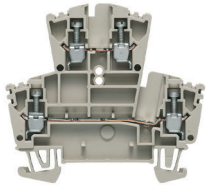
WDK 2.5
