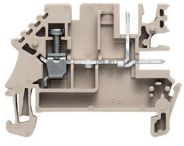
WDU 1.5/BLZ 5.08
