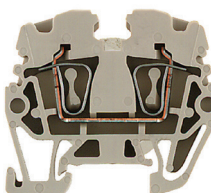
ZDUA 2.5-2
