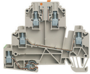
WDK 2.5/TR-DU-PE
